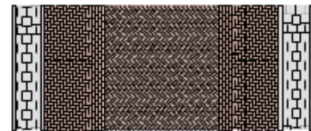
Trottoir Langparkeerzone Rijweg Langparkeerzone Trottoir
